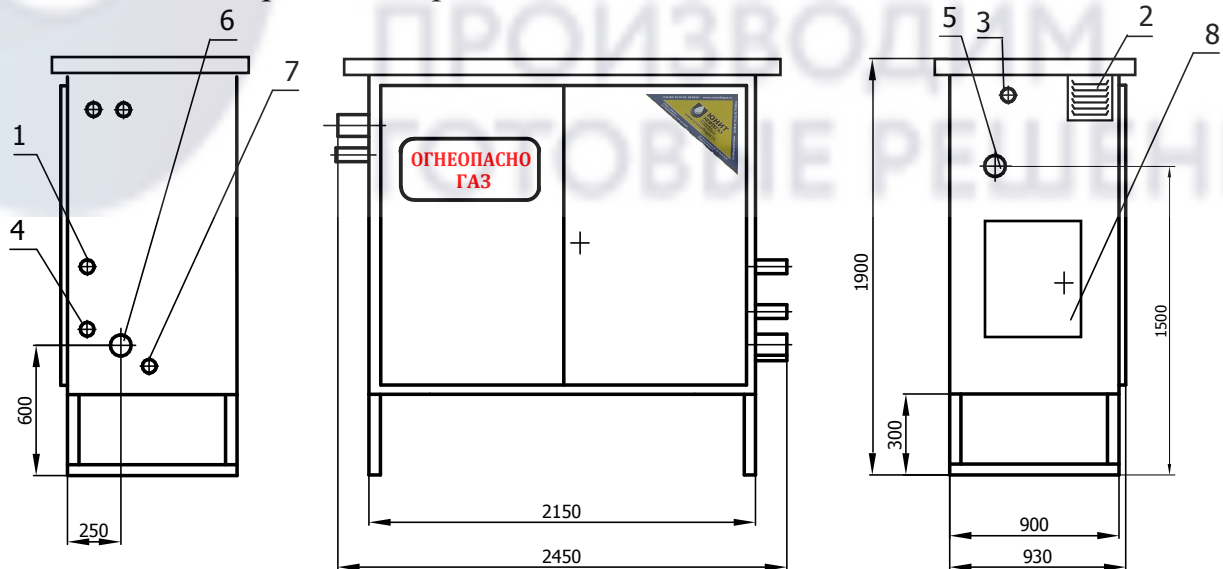
Габаритный чертеж
